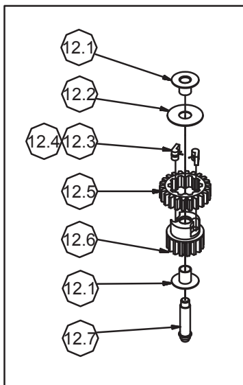
ITEM No. 12 - 775600 / 775650
