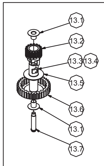
ITEM No. 13 - 775500
